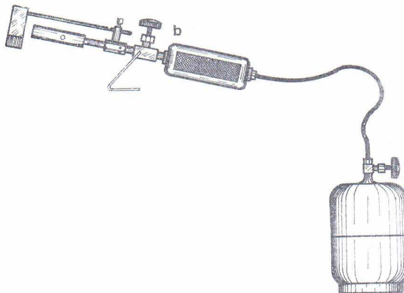
Soldador de cobre con mechero de gas
